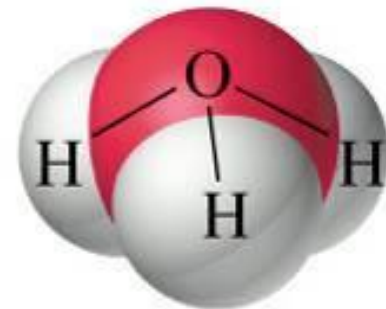
Hydronium ion \text{H}_3\text{O}^+
