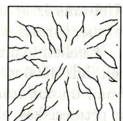
radiālais tīkls
