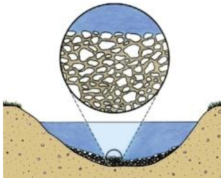
Daudz sedimentu
