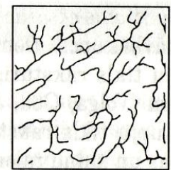
deformētais tīkls
