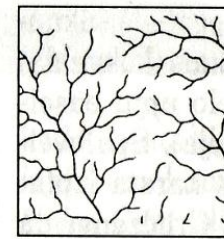
dentritiskais tīkls
