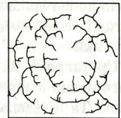
gredzenveida tīkls
