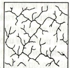
taisnleņķa tīkls
