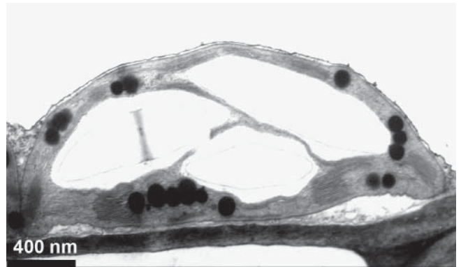
B_11_DD_01_VM2_hloroplasts_2.jpeg
