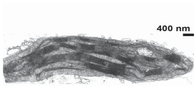
B_11_DD_01_VM2_hloroplasts_4.jpeg
