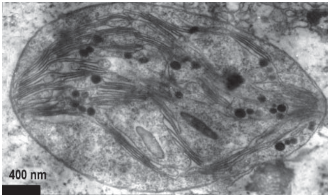
B_11_DD_01_VM2_hloroplasts_1.jpeg
