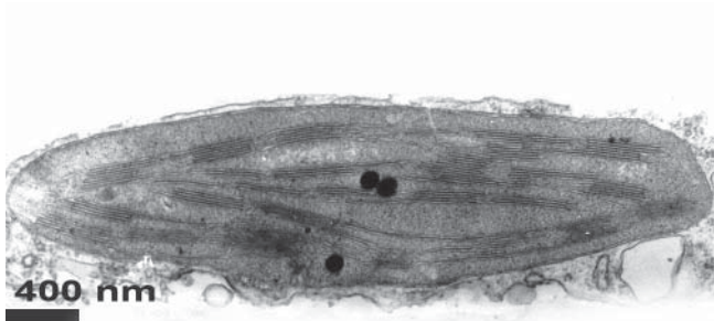
B_11_DD_01_VM2_hloroplasts_3.jpeg
