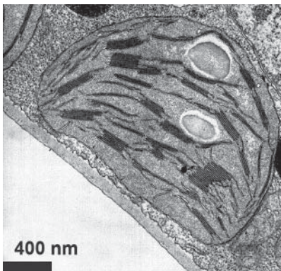
B_11_DD_01_VM2_hloroplasts_5.jpeg
