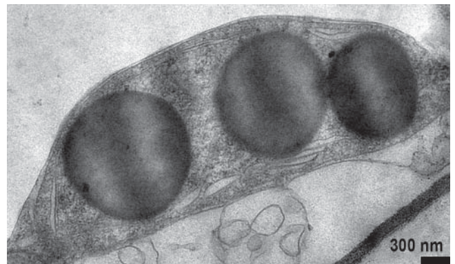
B_11_DD_01_VM2_hloroplasts_6.jpeg
